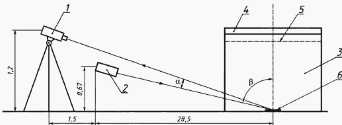
1 — аркомер; 2 — источник света; 3 — дождевальная установка; 4 — шланг; 5 — сетка; 6 — дорожная разметка (Расстояния в метрах)
