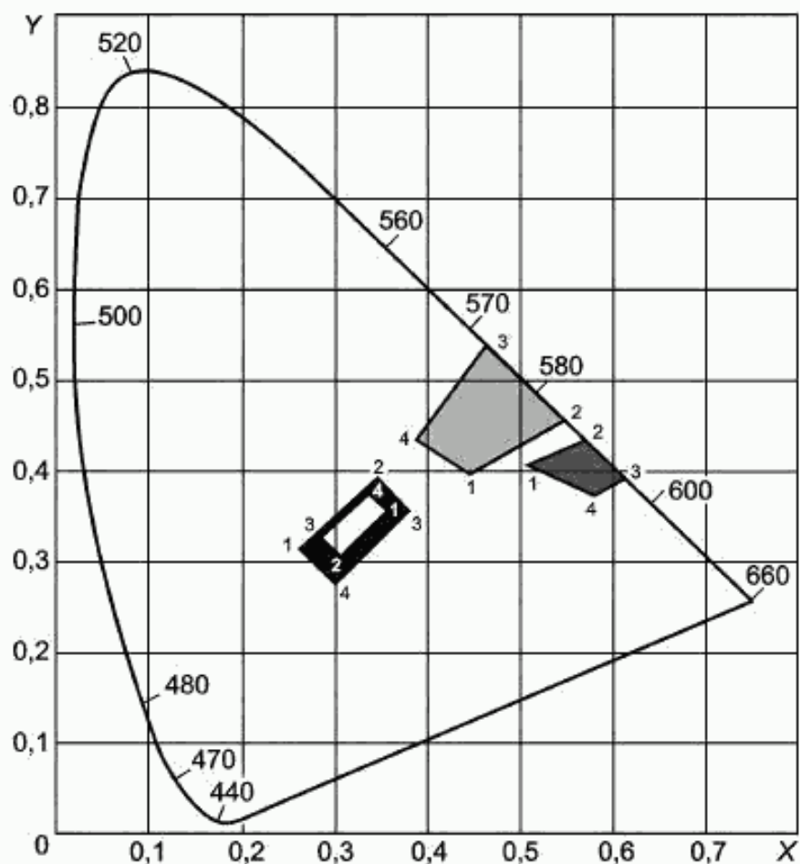
Рисунок В.1 — График цветовой области для дорожной разметки (МКО, 1931)
