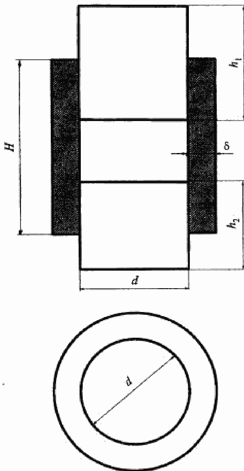
Рисунок 2 — Форма для изготовления образцов
